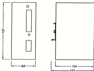
Габаритный чертеж Размеры в мм
